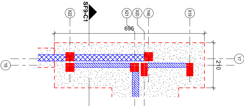
19 SF9 1 : 50
