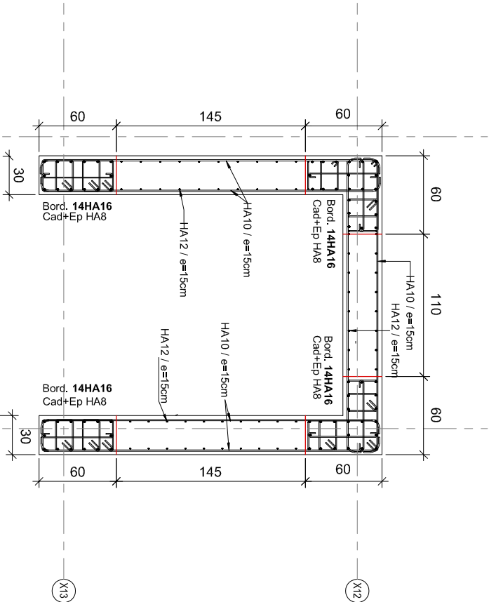
2 V-MC-2 1 : 20
