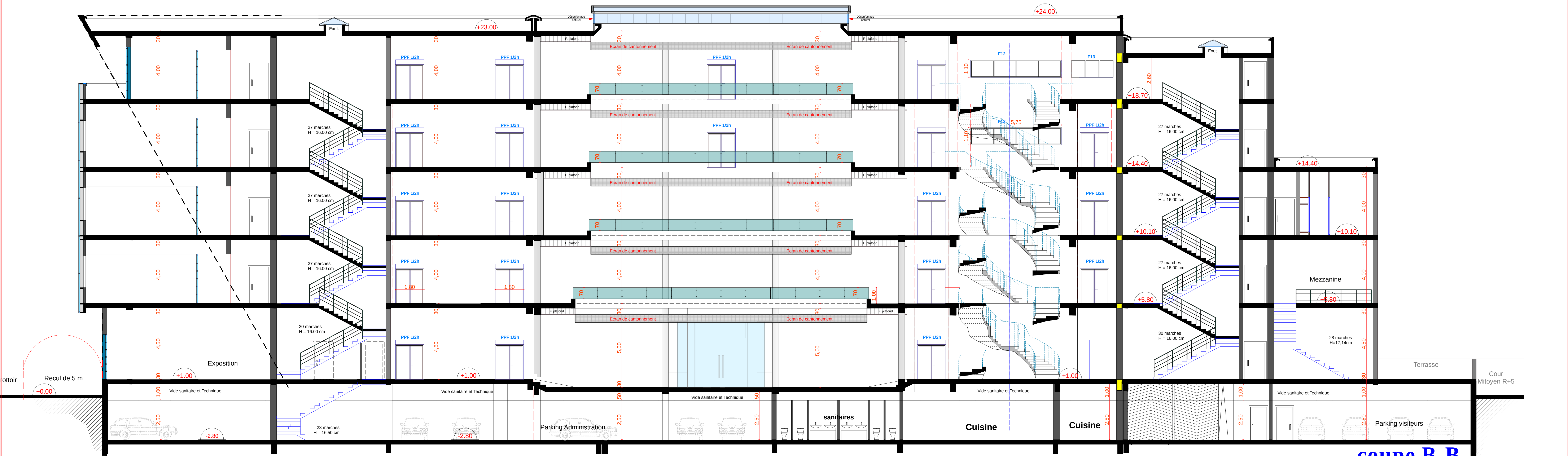
coupe B-B
